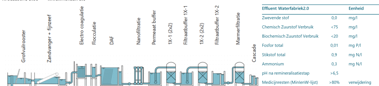
AFBEELDING 5.11 WATERFABRIEK 2.0
