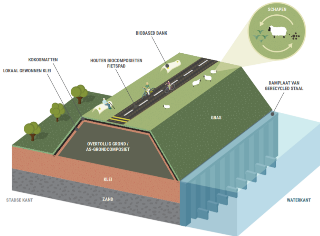
AFBEELDING 5.13 CIRCULAIRE DIJKENBOUW
