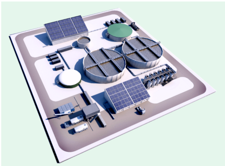
AFBEELDING 5.10 MODULAIRE RIOOLWATERZUIVERINGSINSTALLATIE. BRON: VERDYGO 63
