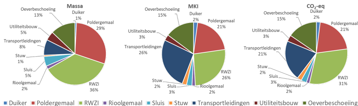
AFBEELDING 4.7 RELATIEVE MASSA, CO 2 -EQ EN MKI VOOR EEN GEMIDDELD WATERSCHAP
